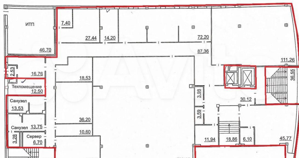
1 ЭТАЖ
